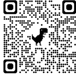
Android
